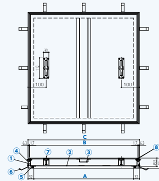
断面図 (ロック無)
