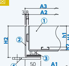
断面図
