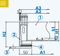
断面図
