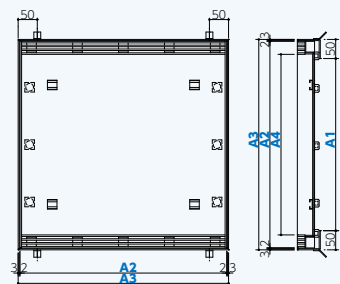
平面図
