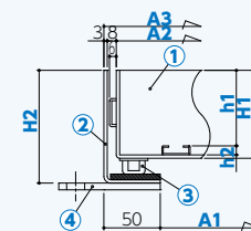
断面図
