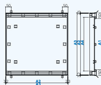
平面図
