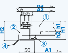
断面図
