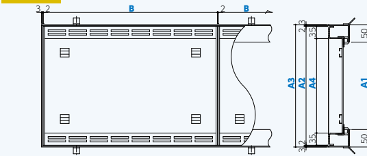
平面図
