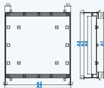
平面図
