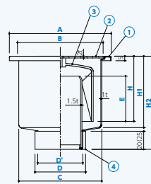
詳細図
