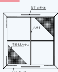
詳細図 平網タイプ
