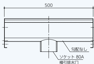
側面図・納まり図
