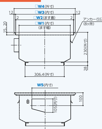
側面図・納まり図
