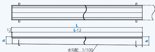
側面図
