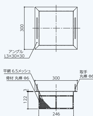
側面図・納まり図
