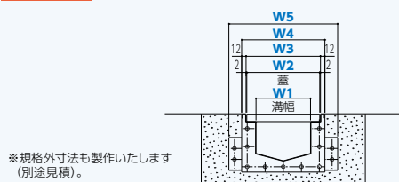
納まり図
