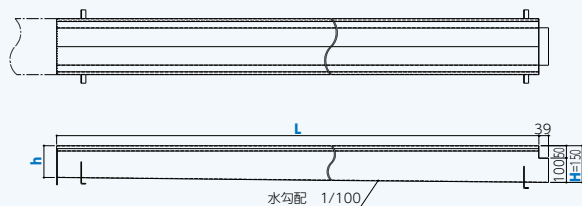
納まり図
