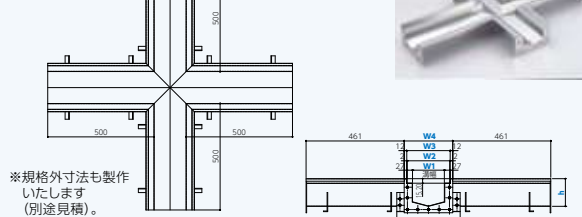
側面図
