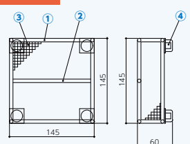
側面図
