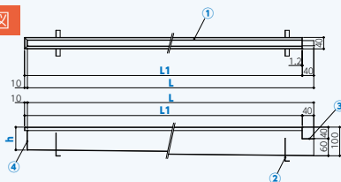
納まり図
