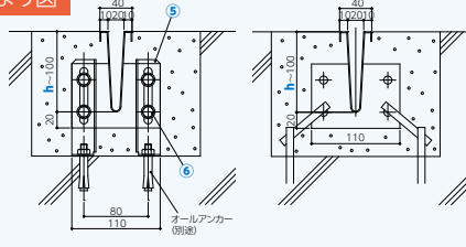
納まり図
