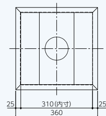
側面図・納まり図
