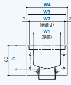
側面図
